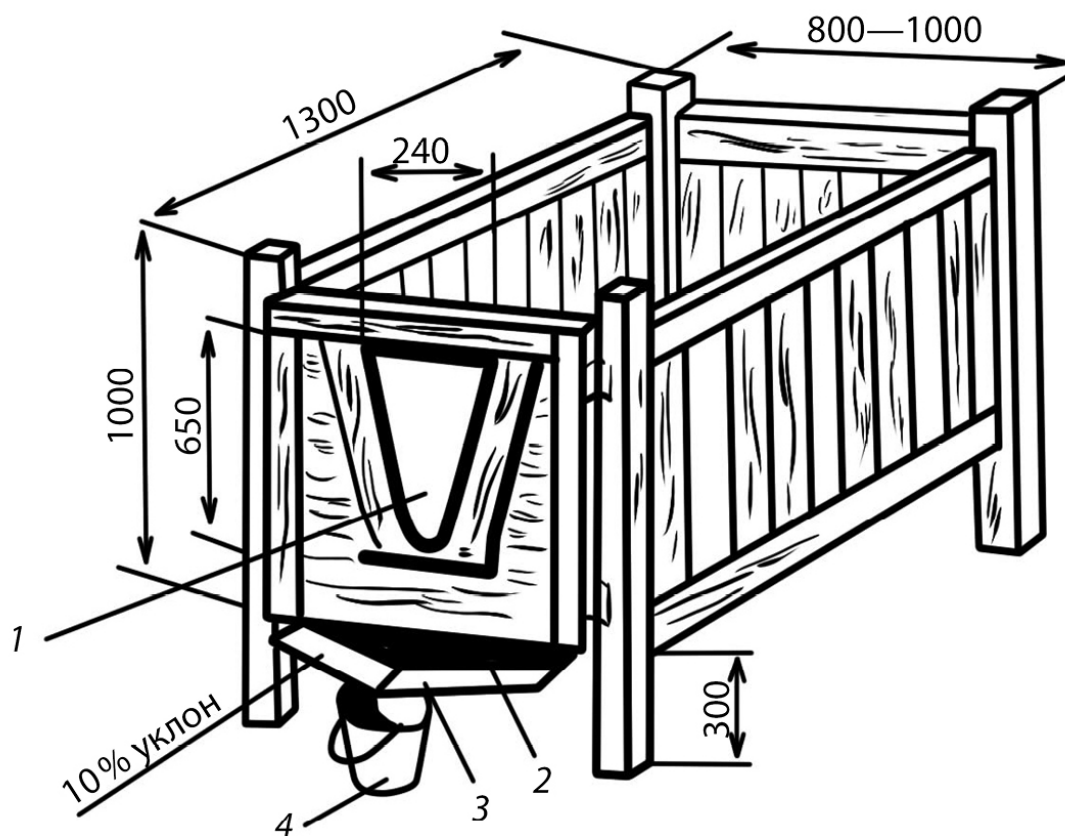
Рис. 3. Клетка для содержания теленка:
